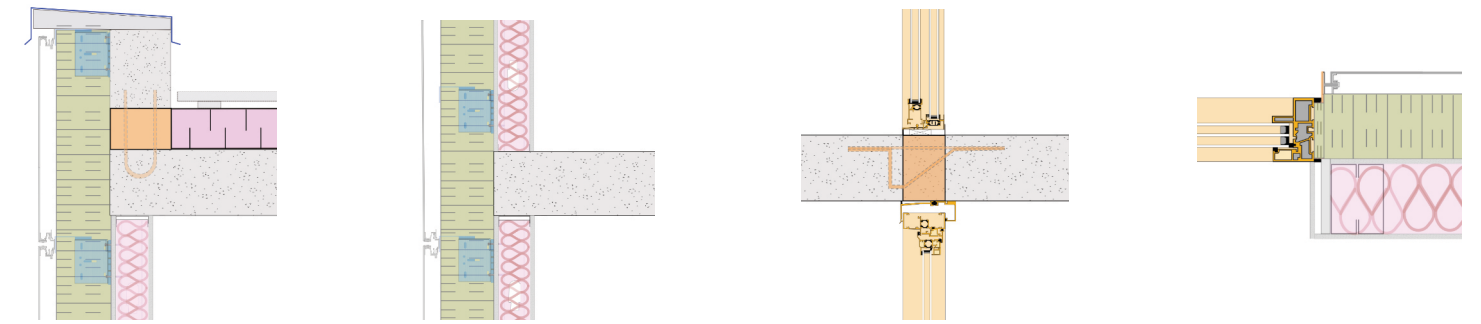
Toiture-mur Plancher intermédiaire Balcon en porte-à-faux Fenêtre-mur
