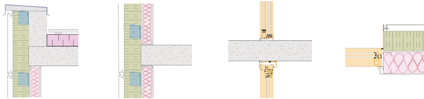
Toiture-mur Plancher intermédiaire Balcon en porte-à-faux Fenêtre-mur
